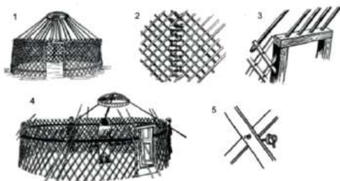
Рисунок 3. – Конструкция юрты и ее установка
