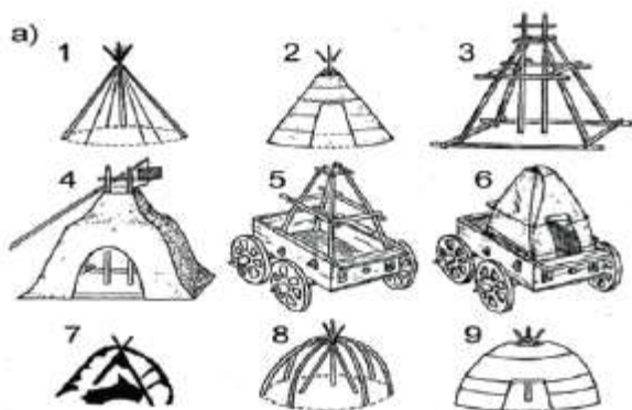
Рисунок 1. – Классификация мобильных сооружений (по С.И. Вайнштейну)
